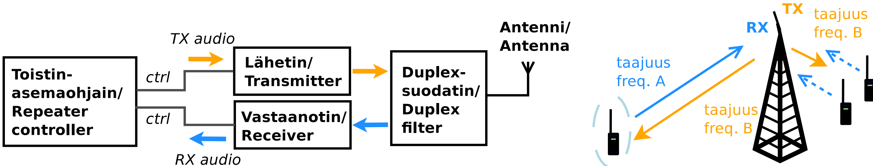
Tyypillisen analogisen taajuusjakoisen (FDD) radioamatööri-toistimen periaate Principle of a typical analog frequency-division duplex (FDD) HAM radio repeater
